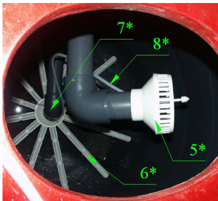
*В зависимости от диаметра бочки фильтра Детализовка «Позиции 2 Таблицы 2» (Обвязки фильтра Kripsol BD 90-125.B) изображена на рисунке 4. Рисунок 4
