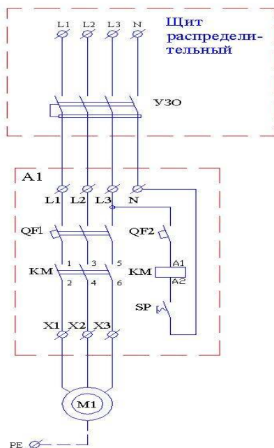
Эл.схема 2
