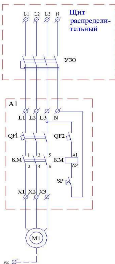
Эл.схема 2
