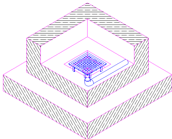
Рисунок 9 (установка сквозь борт)
