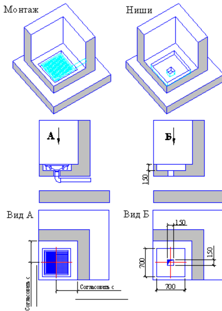
Рисунок 7 (установка платы сквозь борт)
