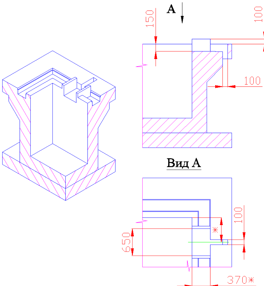
Рисунок 4 (переливной бассейн)
