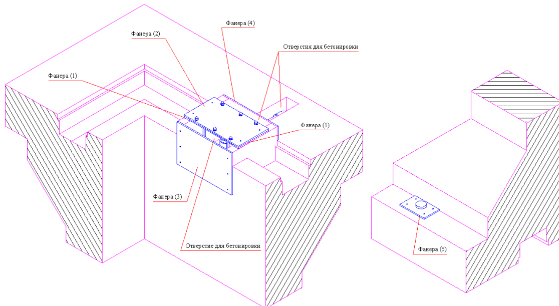
Рисунок 15 (переливной бассейн)
