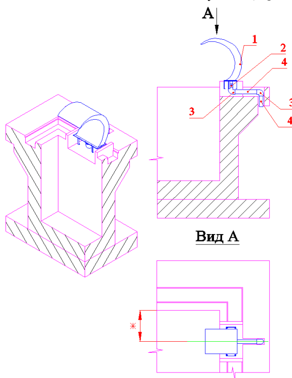
Рисунок 6 (переливной бассейн)
