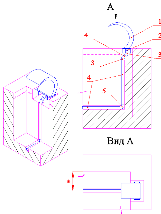
Рисунок 5 (скиммерной бассейн) (прокладка трубопроводов по дну бассейна)
