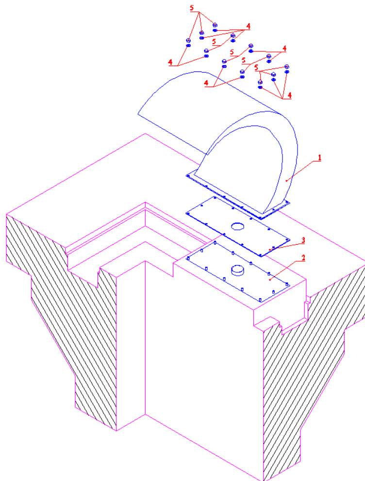
Рисунок 17 (переливной бассейн)
