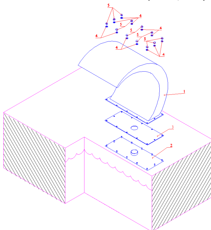
Рисунок 16 (скиммерной бассейн)
