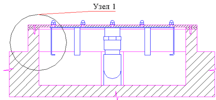
Рисунок 9 (переливной бассейн)
