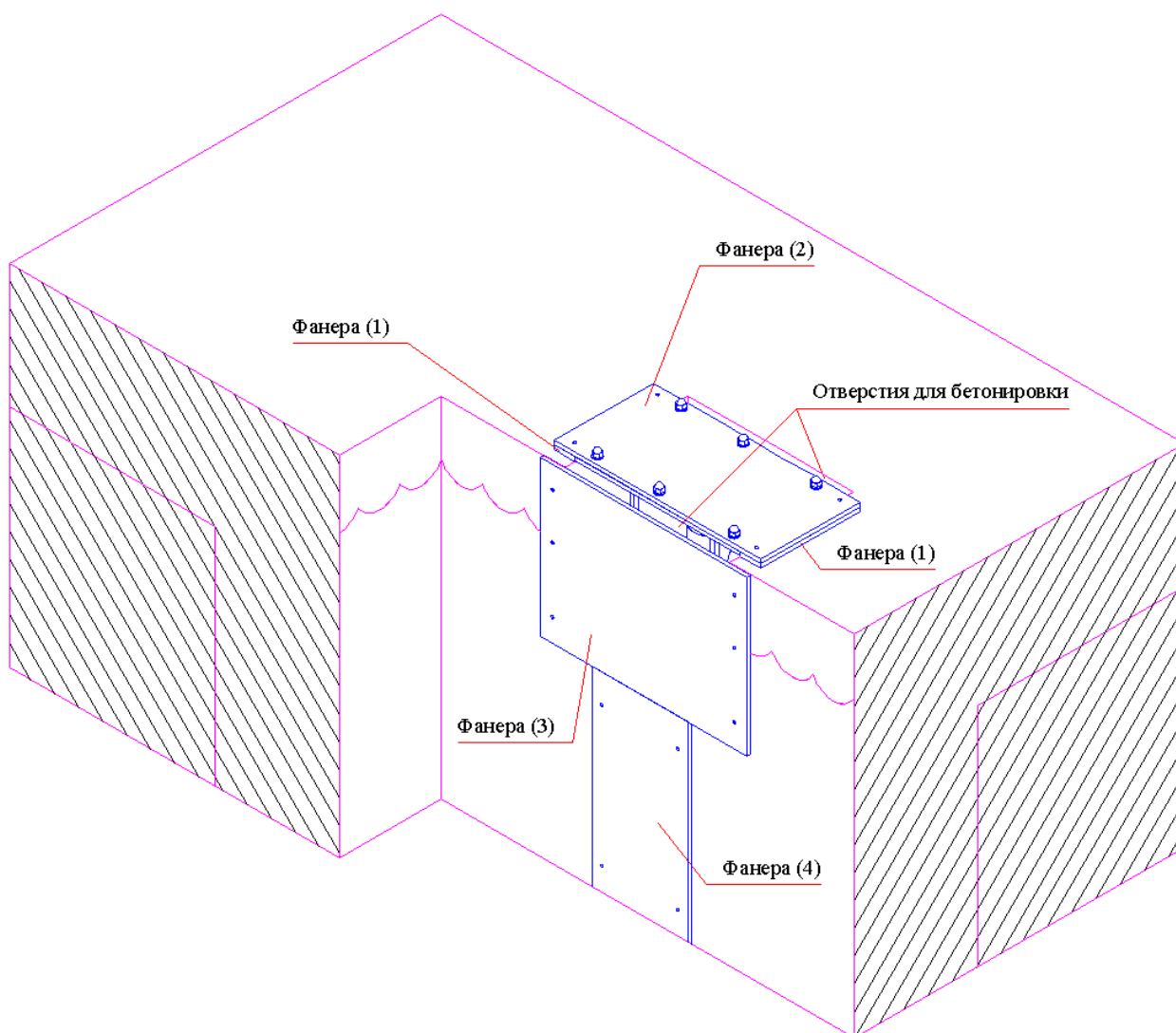
Рисунок 14 (скиммерной бассейн)
