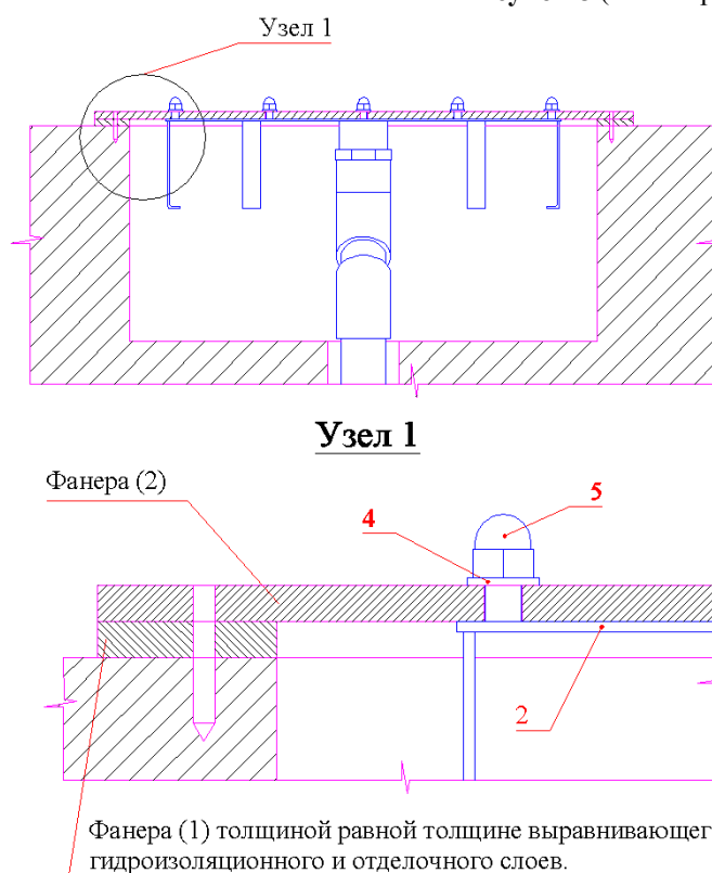
Рисунок 8 (скиммерной бассейн)
