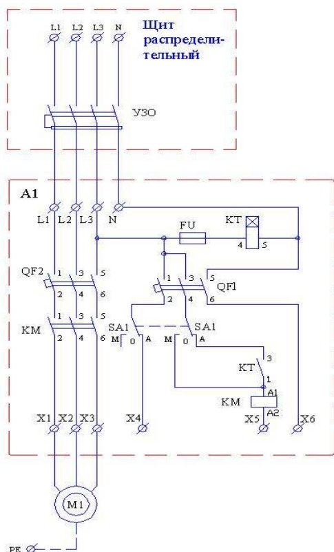
Эл.схема 1
