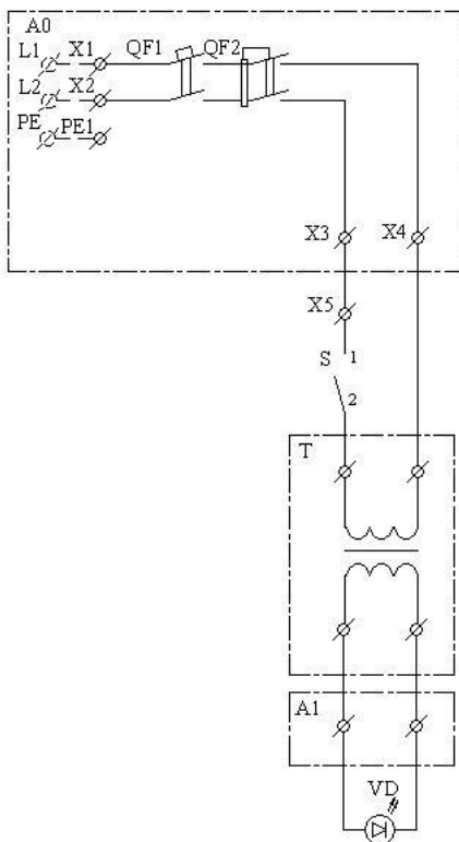
Электрическая схема 1
