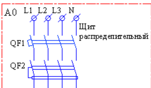
Эл.схема 1
