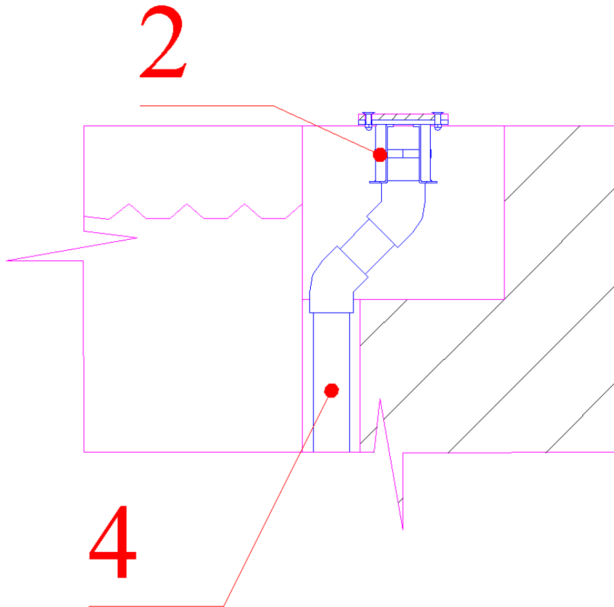
Рисунок 11 (переливной бассейн)
