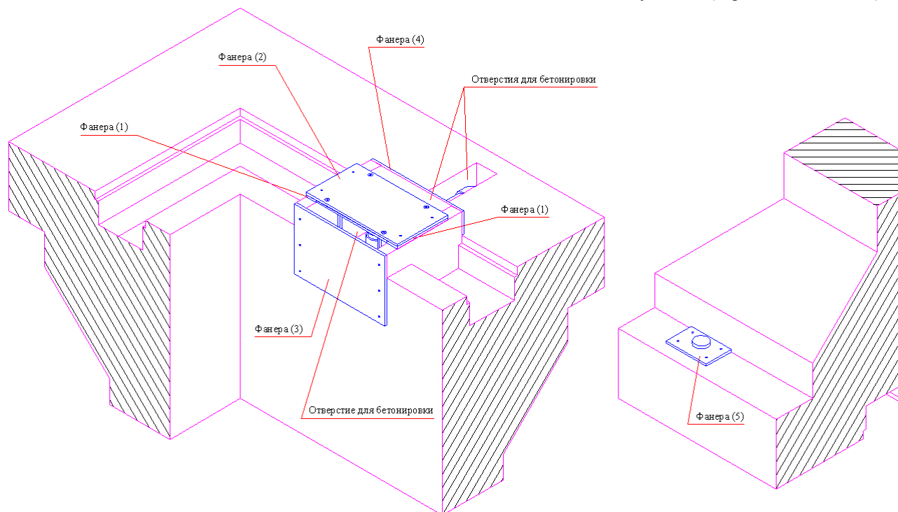
Рисунок 15 (переливной бассейн)
