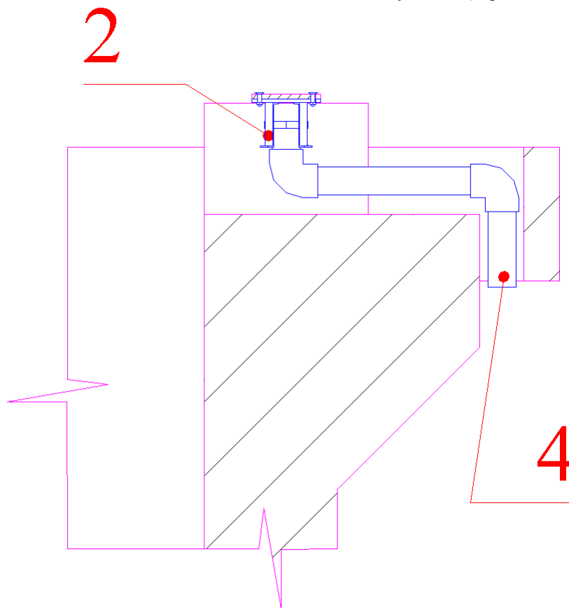
Рисунок 11 (переливной бассейн)
