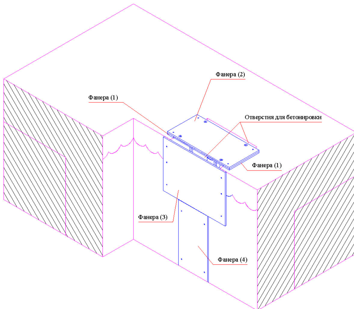
Рисунок 15 (переливной бассейн)
