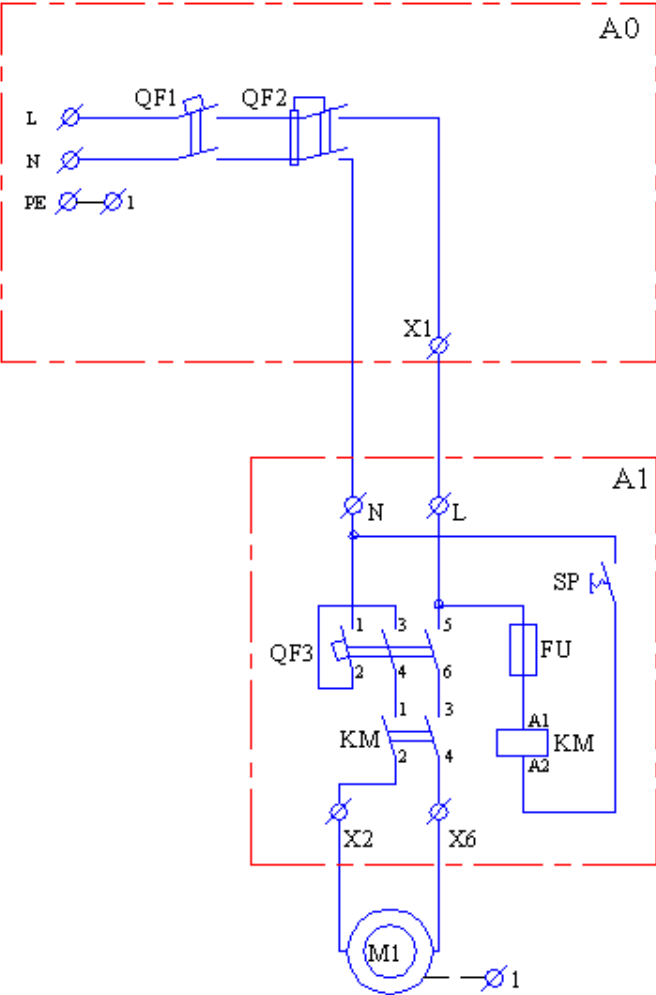
Электрическая схема 1
