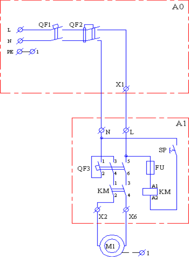
Электрическая схема 1
